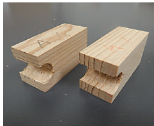
ボルトなどの埋め込み部分から、どれだけ割れが発生しにくいかを確認する試験。 左のように加工し、右のように上下に力がかかる。
