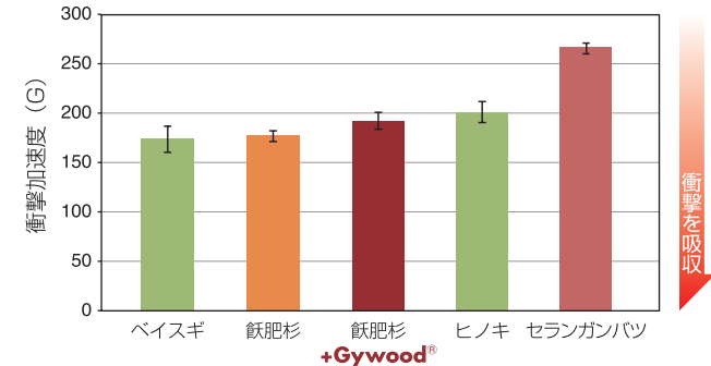
衝撃吸収性比較 あいち産業科学技術総合センターでの試験
