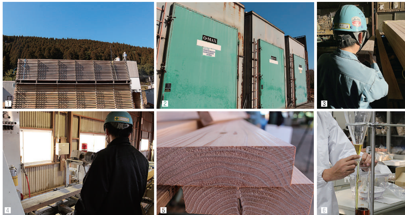
1 天然乾燥中の ObiRED® 2 含水率を整えるために中温の人工乾燥機で仕上げます 3 人の目で1枚1枚丁寧に選別されます 4 製材風景 5 乾燥後4面カンナ削り加工された ObiRED® デッキ材 6 ObiRED® から抽出した精油成分
